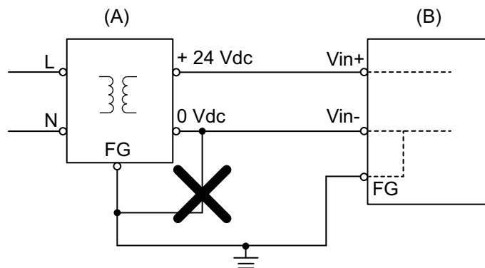
A. DC-Versorgung B. Dieses Produkt
