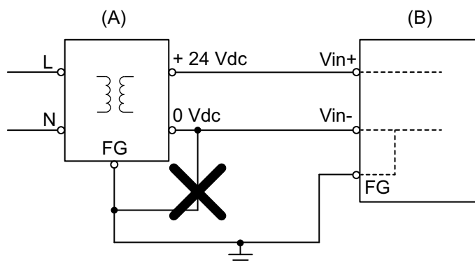
A. Alimentation CC B. Ce produit
