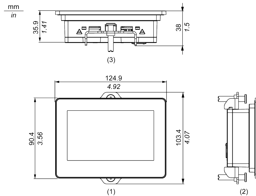
1 正面図
