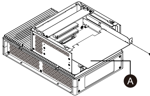
A. Scheda PCI/PCIe
