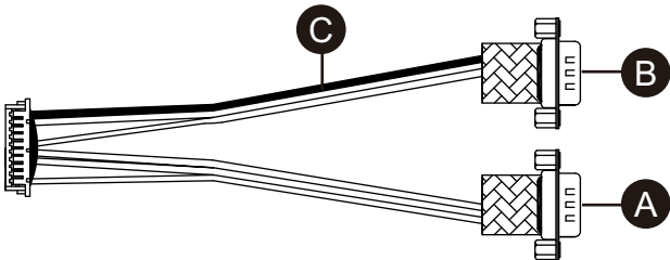
Cavo di interfaccia RS-422
