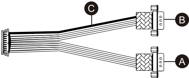
Cavo di interfaccia RS-422
