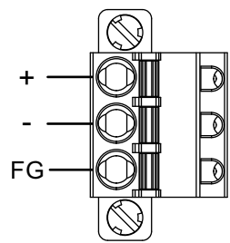
直流电源连接器：弹簧夹型端子块
