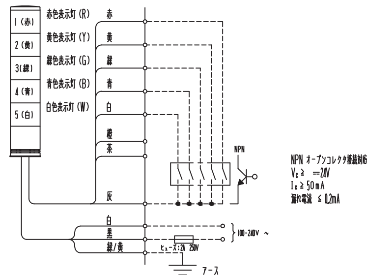
○ 結線図
