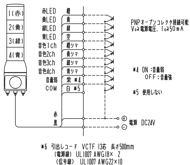
○ 結線図
