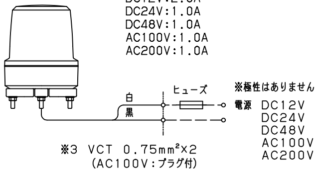
○ 結線図 △
