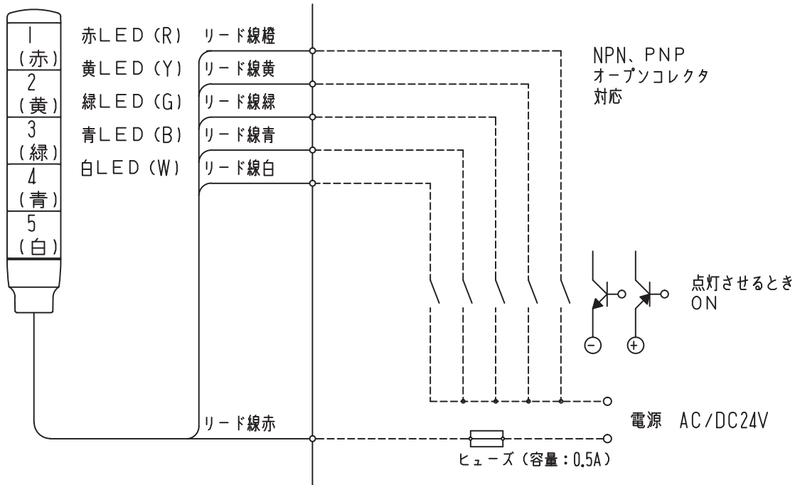
○配線方法
