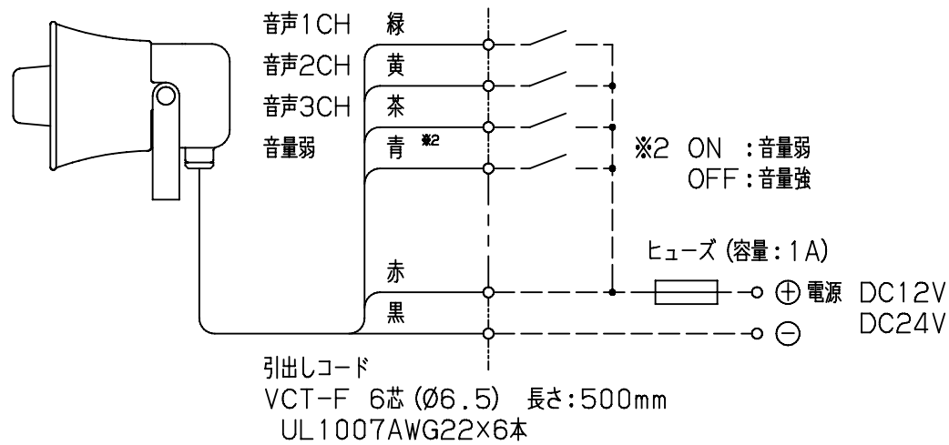
○ 結線図
