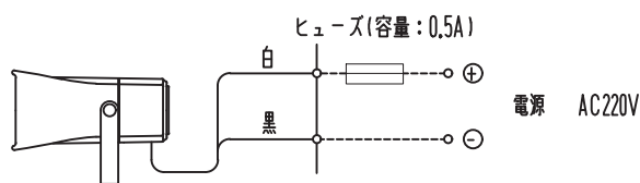
○ 結線図
