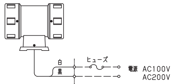
○ 結線図
