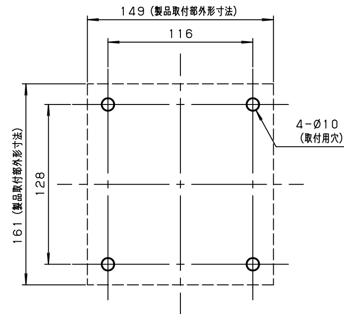
○ 取付穴加工図
