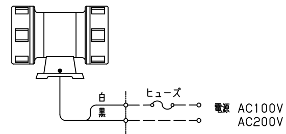
○ 結線図
