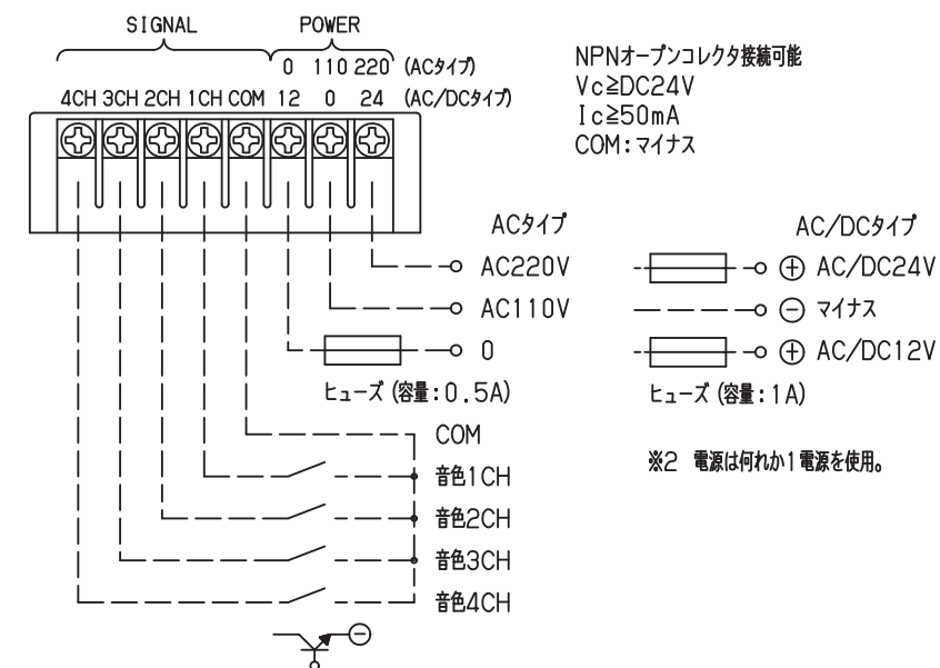
○ 結線図
