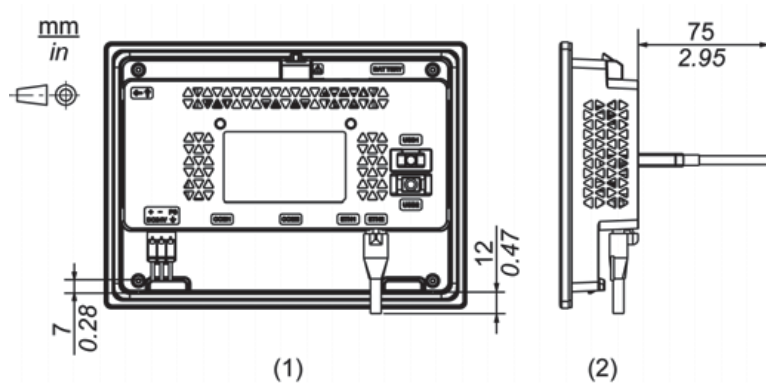
1 背面図
