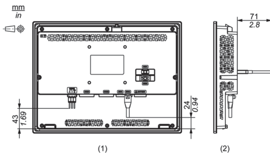
1 背面図
