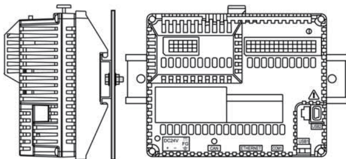
垂直取り付け
