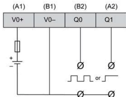
ソース出力（正論理）
