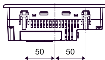
底面図
