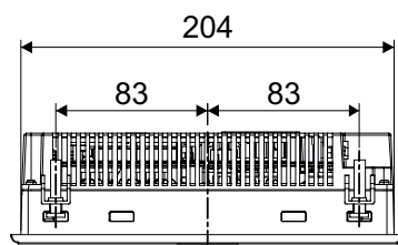
上面図
