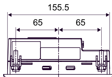
上面図
