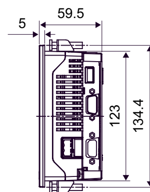
右側面図
