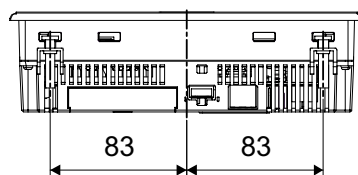
底面図
