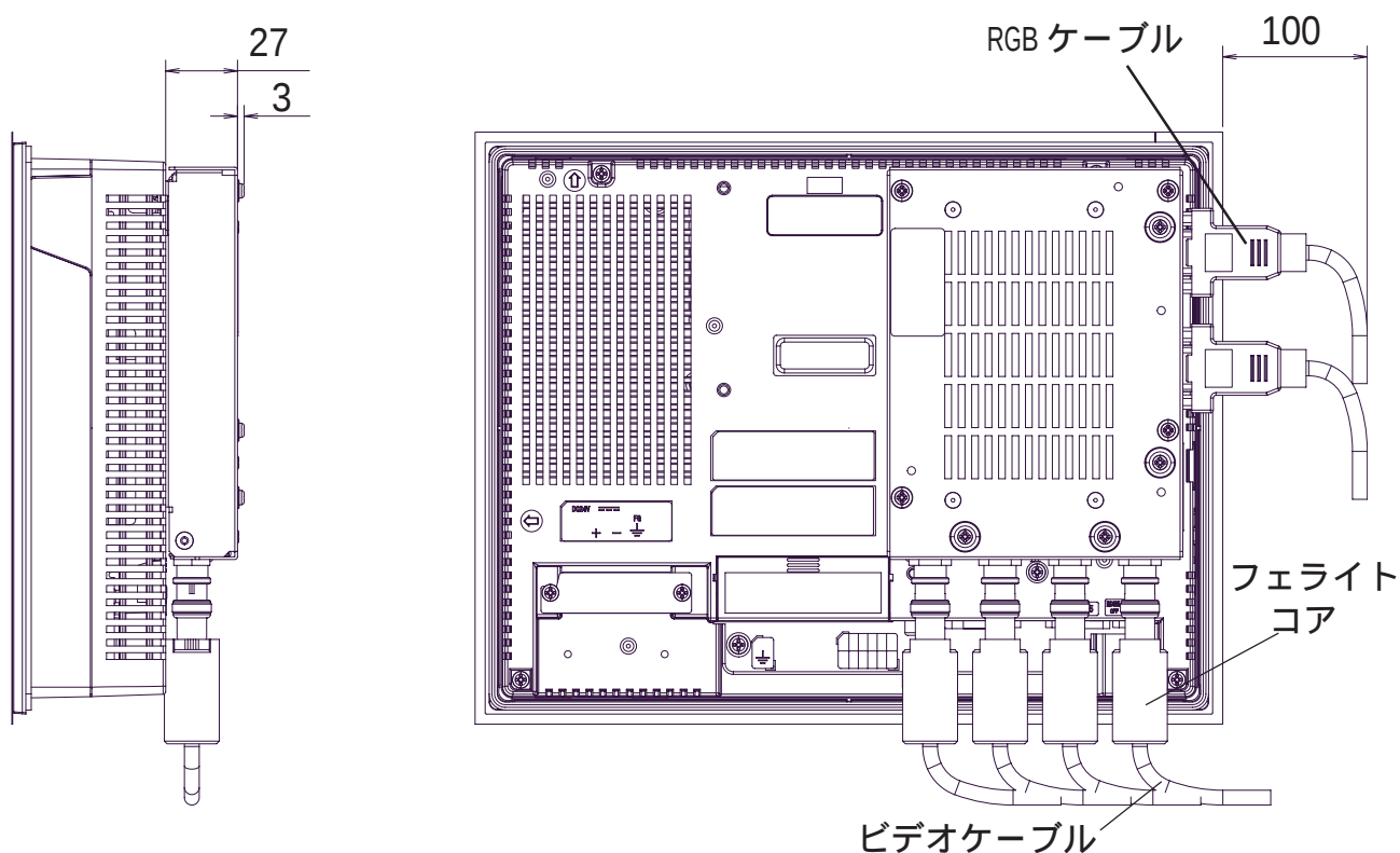
(図は AGP-3550T)
